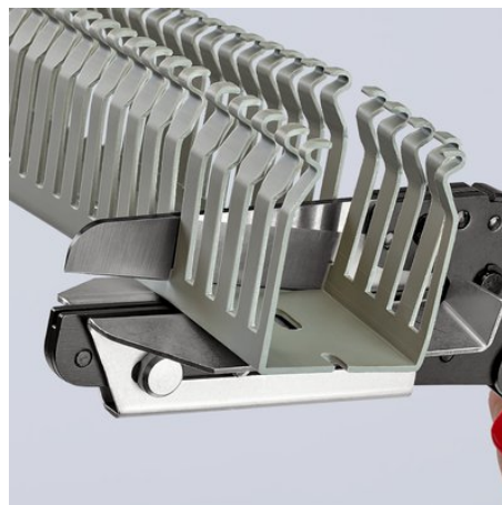
Longueur de la lame 110 mm pour sectionner les goulottes de câbles larges
