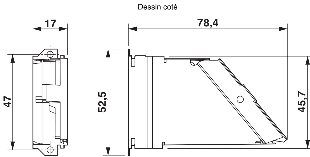
Manchon intérieur CEM SUB-D
