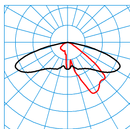
Publisca P1-AB2L/5100-740 6G1S ETDD (CLO end value) TX301496 ■ C0 - C180 ■ C90 - C270 DIN 5040: A30 UTE: 1,00 G CEN Flux Code: 35 74 97 100 100
