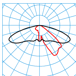
Publisca P1-AB2L/5100-740 6G1S ETDD (CLO initial value) TX300419 ■ C0 - C180 ■ C90 - C270 DIN 5040: A30 UTE: 1,00 G CEN Flux Code: 35 74 97 100 100
