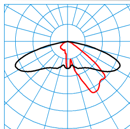
Publisca P1-AB2L/5100-740 6G1S TX047501 ■ C0 - C180 ■ C90 - C270 DIN 5040: A30 UTE: 1,00 G CEN Flux Code: 35 74 97 100 100
