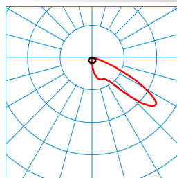
LnStar 70-AM1R/16500-750 6G2C TX051158 ■ C0 - C180 ■ C90 - C270 DIN 5040: A30 UTE: 1,00 l CEN Flux Code: 25 70 98 100 100
