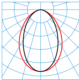
FidescaSD G4 D4 DN 200-940 ETDD TX768075
