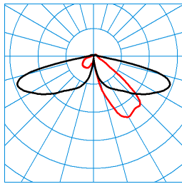
8841LS-Ü 260-AB2L/3200-730 3G2 ET (CLOANFANGSWERT) TX369379 ■ C0 - C180 ■ C90 - C270 DIN 5040: A20 UTE: 0,92 I + 0,08 T CEN Flux Code: 28 63 91 92 100 13 34 62 8
