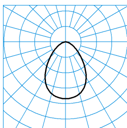
InperiaLP C05 BR22 1800-830 03 + DA-M 03 ■ C0 - C180 TX373078
