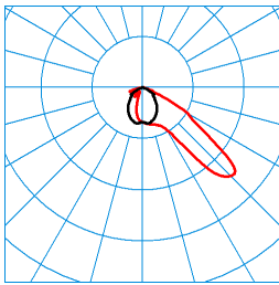
Jovie 50I-AM2L/3200-740 4G1 ETDD TX195490 ■ CO - C180 ■ C90 - C270 DIN 5040: A40 UTE: 1,00 F CEN Flux Code: 47 91 100 100 100
