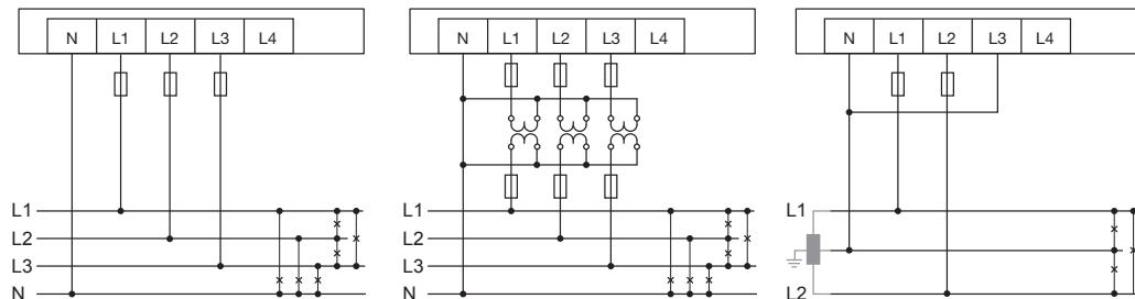
Fig. Exemples de raccordement pour la mesure de la tension dans des "réseaux triphasés à 3 conducteurs" et des "réseaux monophasés à 3 conducteurs". (Variante de raccordement 0, voir page 51)
