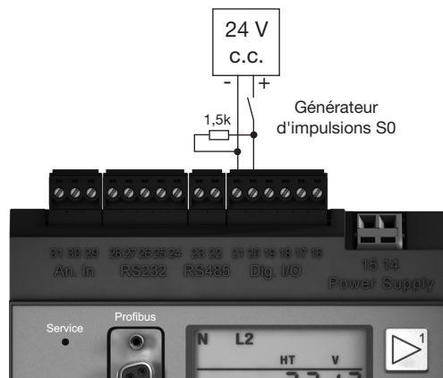
Fig .41.1 UMG604 muni d'entrées pour 24 V. Exemple avec générateur d'impulsions S0.
