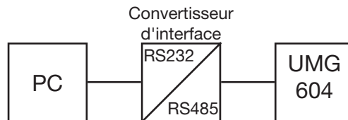
Fig. 13.2. Raccordement d'un UMG604 à un PC par le biais d'un transformateur d'interface.
