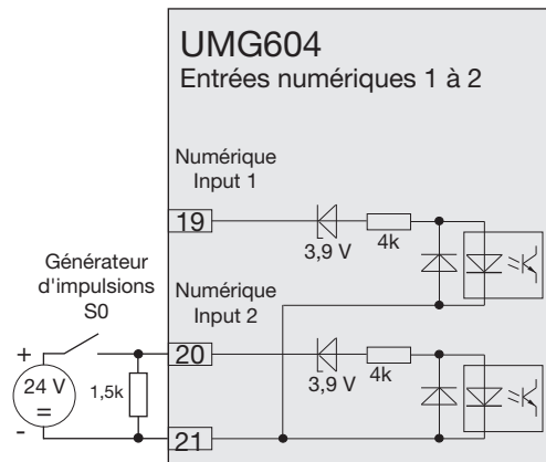
Fi.40.2 UMG604 muni d'entrées pour 24 V. Exemple du raccordement d'un générateur d'impulsions S0 à l'entrée numérique 2.
