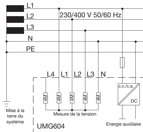
Fig. 15.1 Schéma de principe, UMG604 sur le réseau TN .
