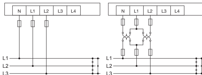
Fig. Exemples de raccordement pour la mesure de la tension dans des "réseaux triphasés à 3 conducteurs". (Variante de raccordement 1, voir page 51)
