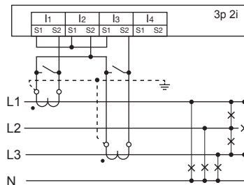
Fig. Mesure de l'intensité, exemple de raccordement pour la variante de raccordement 0 (voir page 50).
