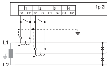
Fig. Mesure de l'intensité sur des systèmes monophasés à 3 conducteurs. Variante de raccordement 0 (voir page 50).
