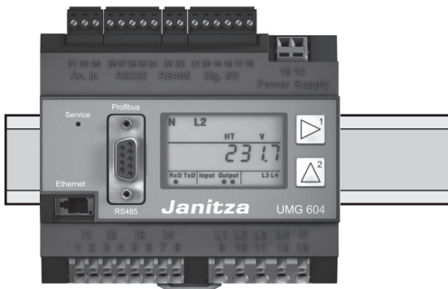
Fig. 22.1 UMG604 sur support profilé selon DIN EN 60715.
