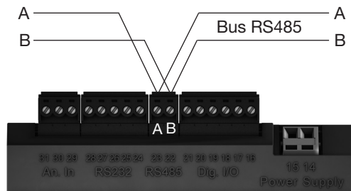
Fig. Interface RS485, contact bipolaire à fiches.
