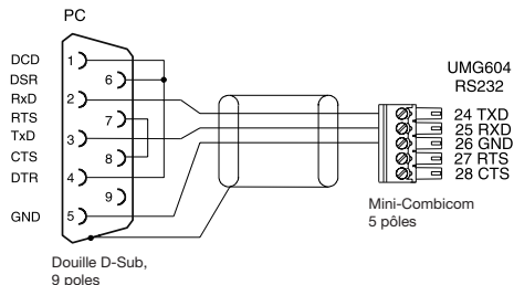
Fig. Affectation des connecteurs pour le câble de raccordement du PC (n° d'art. 08 02 427).
