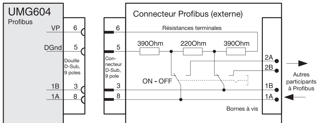
Fig. 37.1 Connecteur Profibus avec résistances de terminaison.
