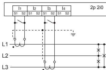
Fig. Mesure de l'intensité, exemple de raccordement pour la variante de raccordement 1 (voir page 50).
