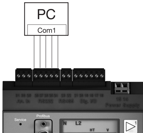
Fig. Exemple de liaison entre un UMG604 et un PC par l'interface RS232.
