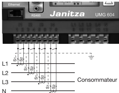
Fig. Exemple de raccordement, mesure d'intensité par transformateur d'intensité.
