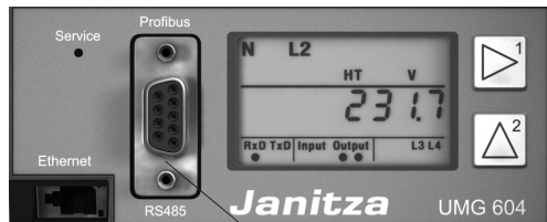
Fig. 36.1 UMG604 avec interface Profibus.
