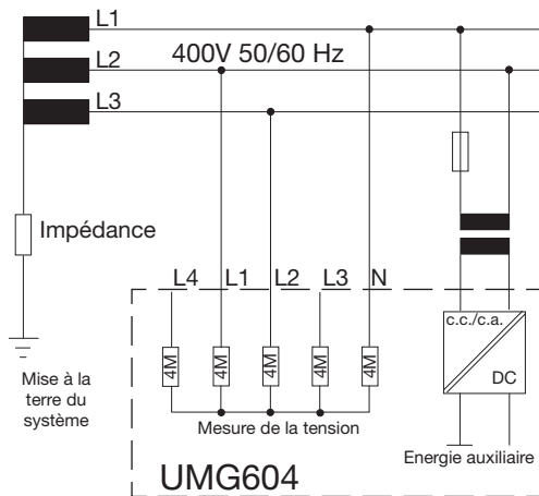
Fig. 17.1. Schéma de principe, UMG604 sur le réseau IT sans N.
