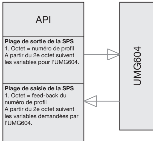
Fig. 54.1 Schéma-bloc pour l'échange de données entre SPS et UMG604.
