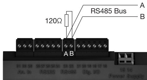
Fig. Interface RS485, contact bipolaire à fiches avec résistance de terminaison (n° d'art. 52.00.008).
