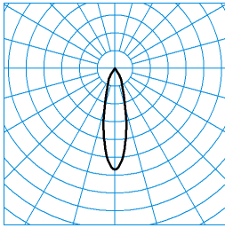
E-Line 7751 B.VEO RFS-MF-c 05 20-BC J24 ET L37 01 ■ C0 - C180 TX095435 DIN 5040: A80 UTE: 0,82 A CEN Flux Code: 100 100 100 100 82
