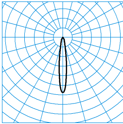
E-Line 7751 B.VEO RFS-SP 05 20-BC J24 ET L37 01 ■ C0 - C180 TX095434 DIN 5040: A80 UTE: 0,81 A CEN Flux Code: 100 100 100 100 81
