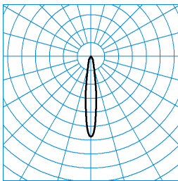
E-Line 7751 B.VEO RFS-SP-c 05 20-BC J24 ET L37 01 ■ C0 - C180 TX095633 DIN 5040: A80 UTE: 0,81 A CEN Flux Code: 100 100 100 100 81
