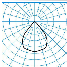
SNS RC5-HR1XFL-14-840 ■ C0 - C180
