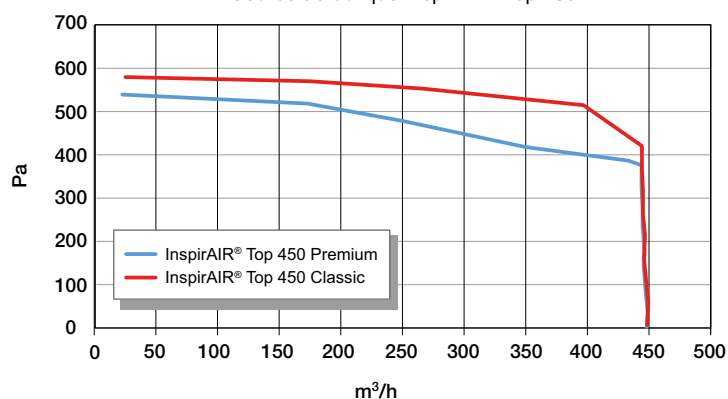
Courbe aéraulique InspirAIR® Top 450
