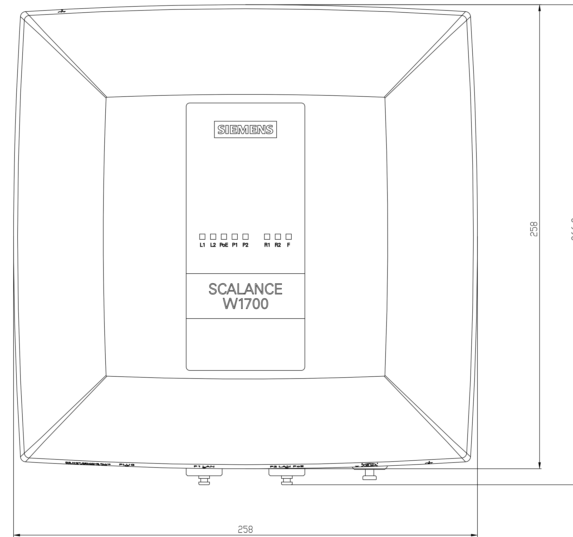
Vorne / Front
