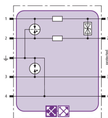
Schéma de principe du circuit BXT ML2 BD HFS 5
