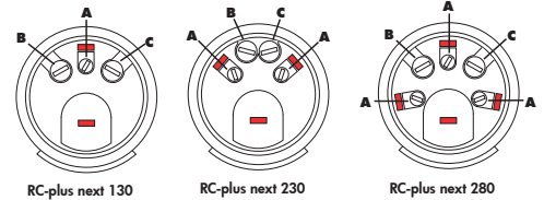
A Portée B Temporisation C Seuil d'enclenchement ■ LED
