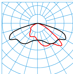
Jovie 70-AB7L-LRA/16500-730 24G1 ET TX076478 ■ C0 - C180 ■ C90 - C270 DIN 5040: A30 UTE: 1,00 G CEN Flux Code: 35 73 97 100 100
