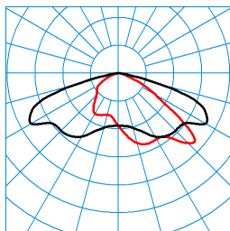
Jovie 70-AB7L-LRA/16500-730 24G1 ET (CLO initial value) TX301291 ■ C0 - C180 ■ C90 - C270 DIN 5040: A30 UTE: 1,00 G CEN Flux Code: 35 73 97 100 100
