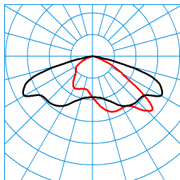
Jovie 70-AB7L-LRA/16500-730 24G1 ET (CLO end value) TX300193 ■ C0 - C180 ■ C90 - C270 DIN 5040: A30 UTE: 1,00 G CEN Flux Code: 35 73 97 100 100
