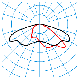
Jovie 70-AB7L-LRA/18000-740 18G1 ET (CLO end value) TX301893 ■ C0 - C180 ■ C90 - C270 DIN 5040: A30 UTE: 1,00 G CEN Flux Code: 35 72 97 100 100
