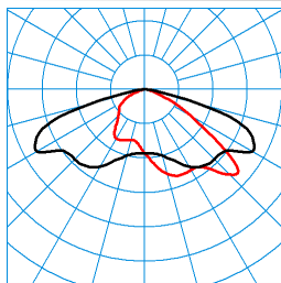
Jovie 70-AB7L-LRA/18000-740 18G1 ET TX068634 ■ C0 - C180 ■ C90 - C270 DIN 5040: A30 UTE: 1,00 G CEN Flux Code: 35 72 97 100 100
