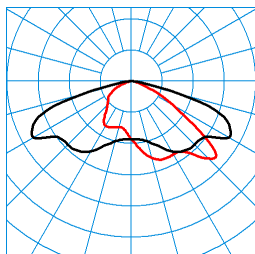
Jovie 70-AB7L-LRA/18000-740 18G1 ET (CLO initial value) TX300430 ■ C0 - C180 ■ C90 - C270 DIN 5040: A30 UTE: 1,00 G CEN Flux Code: 35 72 97 100 100
