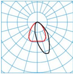
ELINE LAN40-110 ML 865 L150 2 50 ■ C0 - C180
