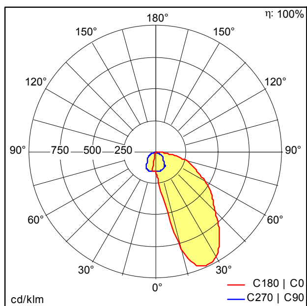
D34983AA_TECTON_C_LED7400-840_L2000_WW_EVG_SR.Idt
