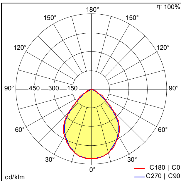
D43600AA_CLEVO_MSC_2700-840_L1280_LDO_WH_WHM.Idt
