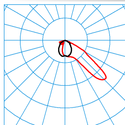
Jovie 50I-AM2L-LRA/3200-730 4G1 ET TX195505 ■ C0 - C180 ■ C90 - C270 DIN 5040: A40 UTE: 1,00 F CEN Flux Code: 47 91 100 100 100
