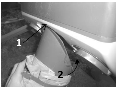
Cliper les piquages en respectant l'ordre 1 puis 2 (cuisine D125, sanitaires D80). Montage à 90° (8) ou en ligne (8bis)
