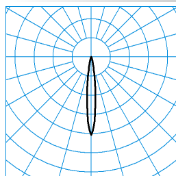
Faciella 08 RE1L/120-blue 1G1 TX045285 ■ C0 - C180 DIN 5040: A80 UTE: 0,99 A CEN Flux Code: 96 100 100 100 99
