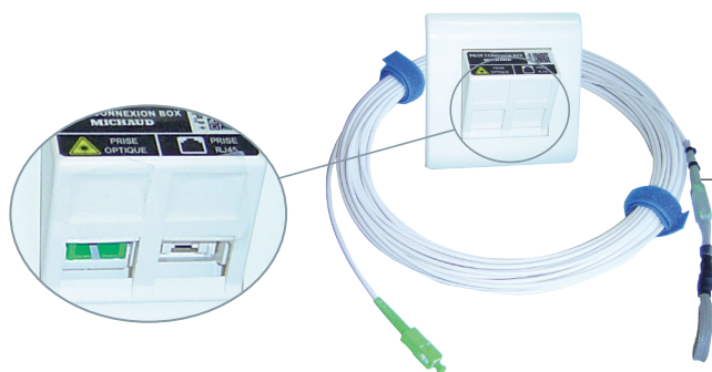
Kit prise box FTTH + jarretière (Q182)
