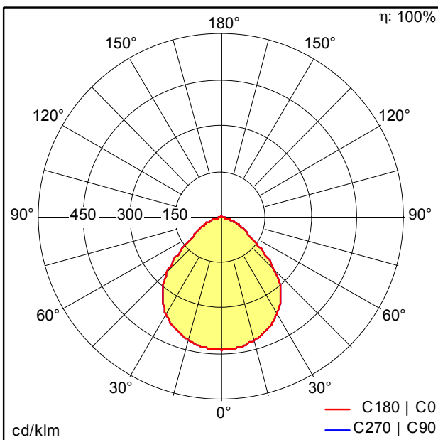
D37457AA_ONDA2_A_LRO_D1150_LED16000-840.idt
