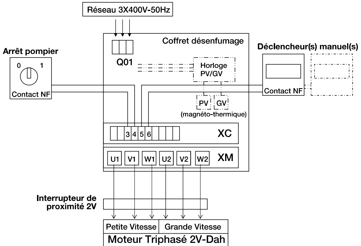
Schéma de câblage simplifié
