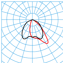
Jovie 70I-AM3L-LR/18000-740 18G1 ET (CLO end value) TX301737 ■ C0 - C180 ■ C90 - C270 DIN 5040: A50 UTE: 1,00 D CEN Flux Code: 59 89 100 100 100
