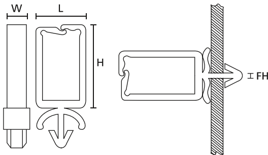
Clip série WPC
