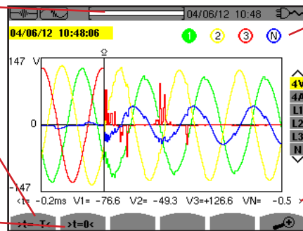
Figure 41 : exemple d'affichage des transitoires sous forme de courbes en branchement triphasé 5 fils
