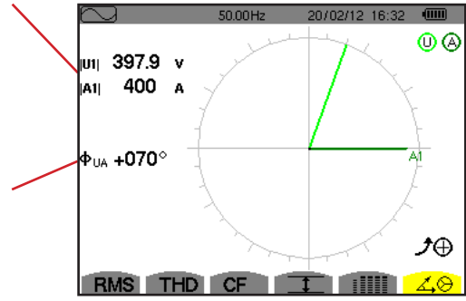
Figure 84 : l'écran d'affichage du diagramme de Fresnel en Diphase 2 fils
