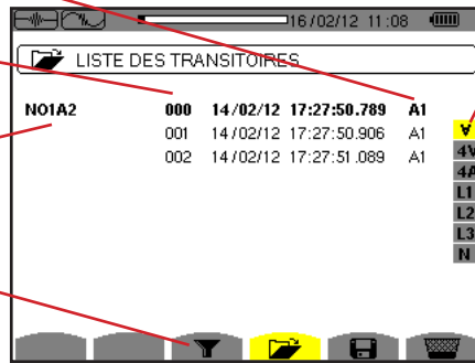
Figure 40 : l'écran Liste des transitoires dans le cas d'un montage triphasé 5 fils
