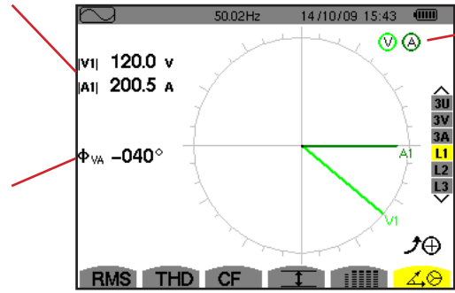
Figure 83 : l'écran d'affichage du diagramme de Fresnel en L1
