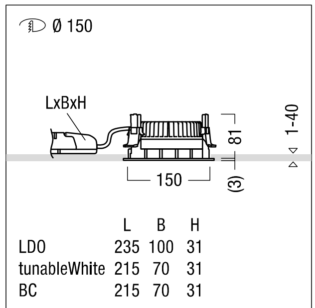
ZS_PAIF_M_R150L_LED_TL.wmf
