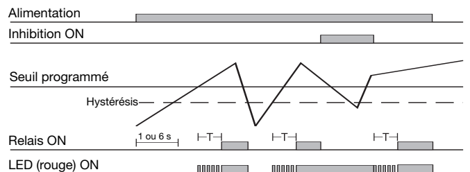
Maxi tension - inhibition activé - Relais normalement désactivé
