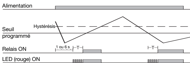
Mini tension - Relais normalement désactivé
