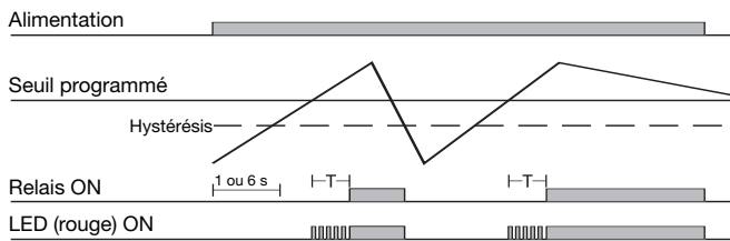
Maxi tension - Relais normalement désactivé
