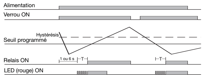
Mini tension - verrou activé - Relais normalement désactivé
