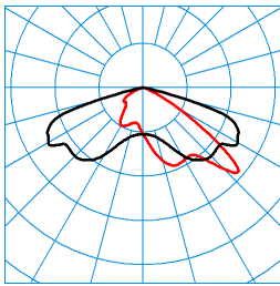
LIQ 70-AB7L-SLR2/6800-740 8G1S TX122204
