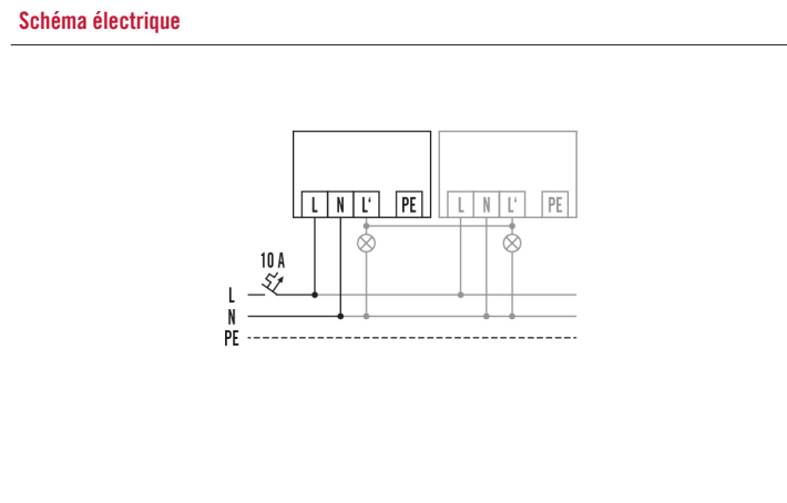
Raccordement optionnel de luminaires automatiques en parallèle
