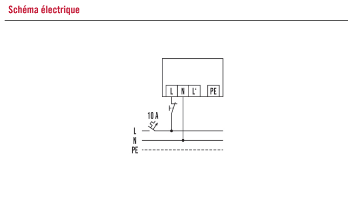
Raccordement avec commande optionnelle par poussoir.
