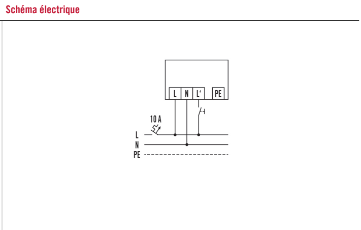
Raccordement standard avec fonction d'éclairage permanent commandée par interrupteur externe.
