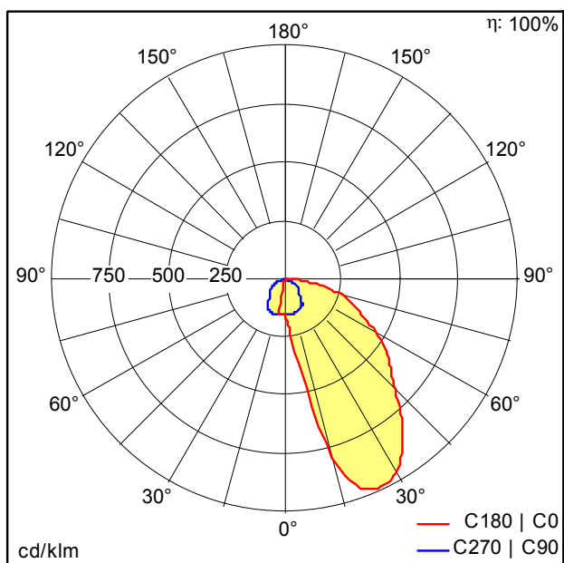
D34983AA_TECTON_C_LED5500-840_L1500_WW_LDE_BK.Idt
