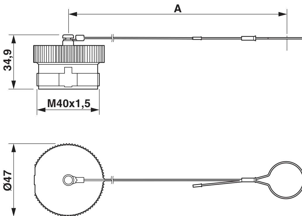
Dessin coté
