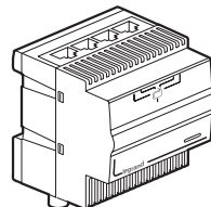
Répartiteur amplificateur TV-SAT sur RJ 4 sorties RJ 45
