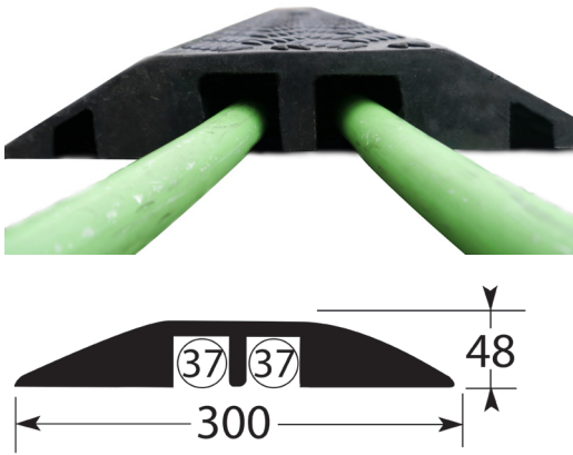
Pont véhicule 37-2
