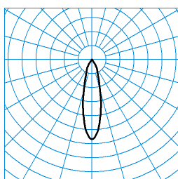
E-Line 7751 B.VEO RFS-MF 05 30-EW J10 ET L37 05 ■ C0 - C180 TX095371
