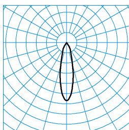
E-Line 7751 B.VEO RFS-MF-c 05 30-EW J10 ET L37 05 ■ C0 - C180 TX095470
