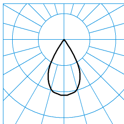
E-Line 7751 B.VEO RFS-VFL 05 30-EW J10 ET L37 05 ■ C0 - C180 TX095767
