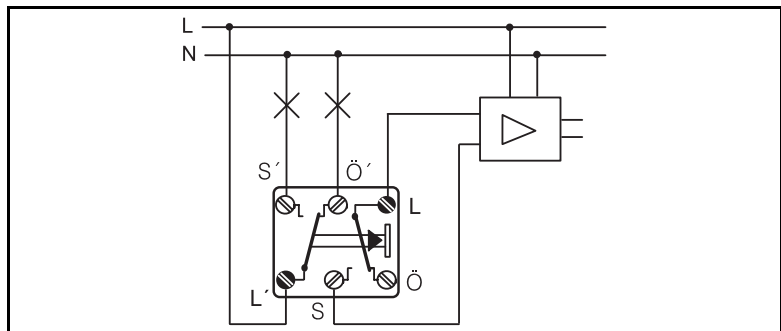
Schémas de raccordement 539 EU
