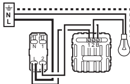
En va-et-vient
