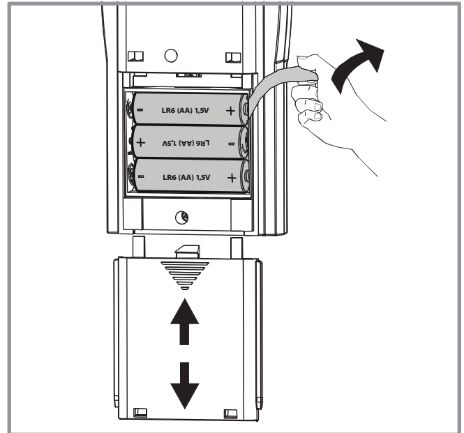
figure 6 - Alimentation de la centrale ambiance
