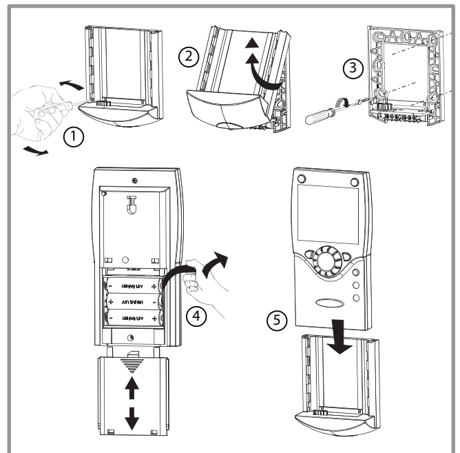
figure 9 - Montage avec socle
