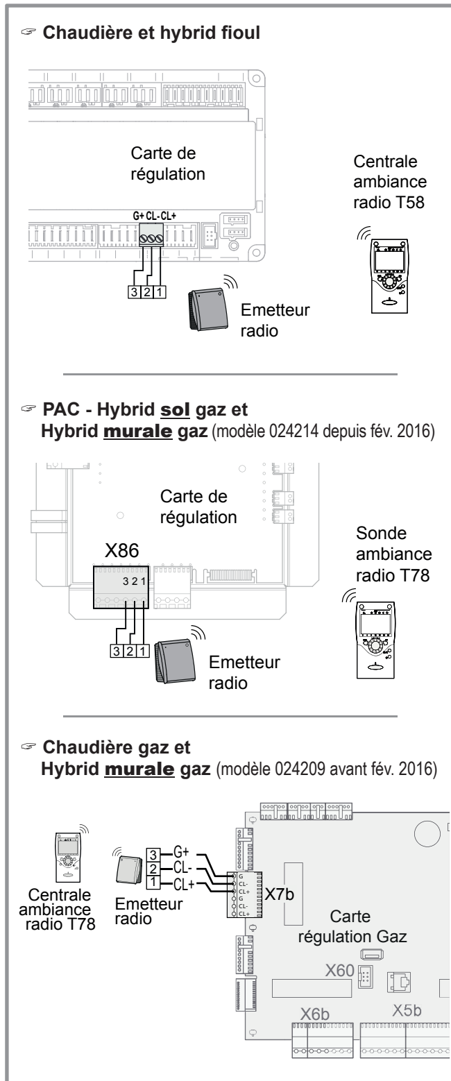
figure 4 - Raccordement de l'émetteur (selon modèle)
