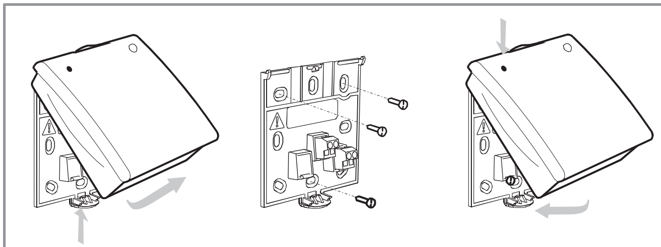
figure 3 - Montage de l'émetteur radio
