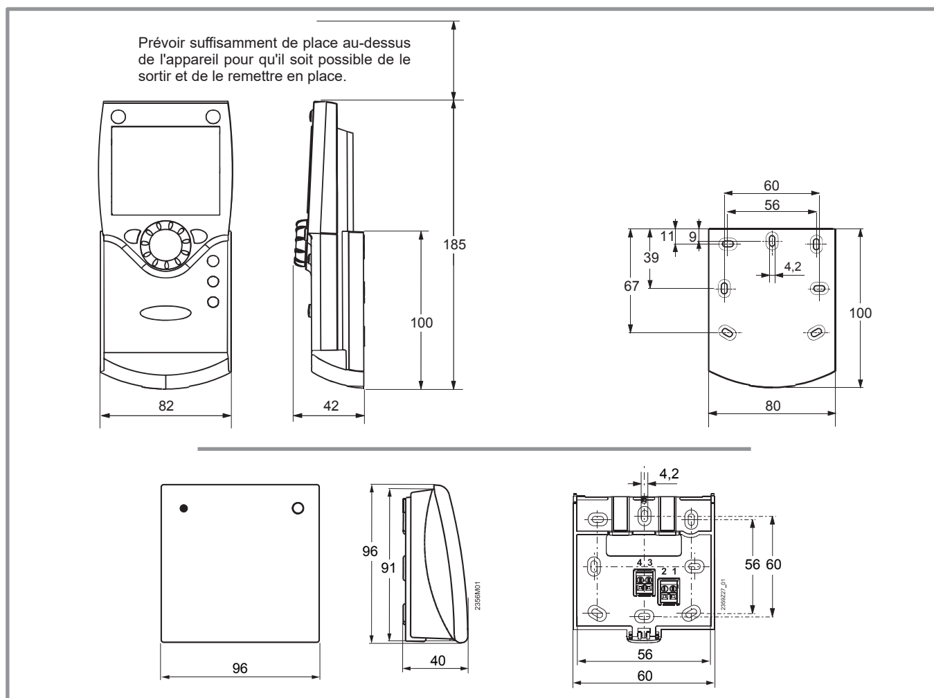
figure 2 - Dimensions en mm
