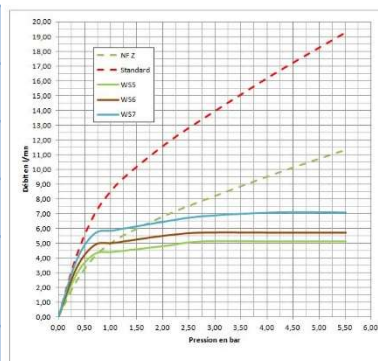
Courbe débit en fonction de la pression et comparaison entre les mousseurs NSF EPA WaterSense (WS 5, 6 ou 7), un NF classe Z et un mousseur standard
