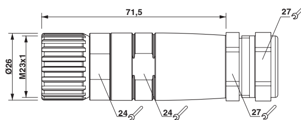
Dessin coté
