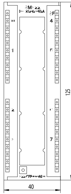
Vorne / Front
