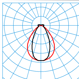
Tugra 18 PN 64-840 ETDD PC LV C2 TX306759
