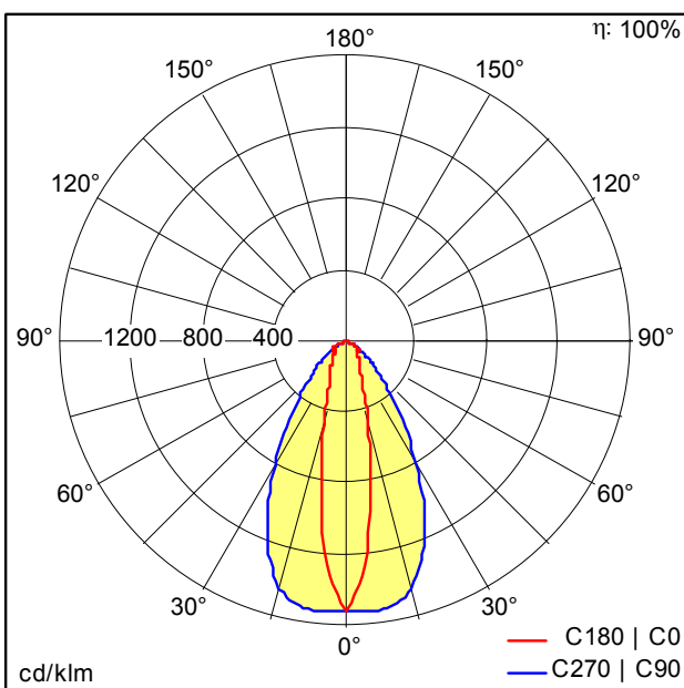
D43653AA_TECTON_C_LED3700-840_L1000_NB_LDE_WH.Idt
