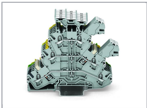
Module de fiche de contrôle type L, ici placé dans une borne à trois étages
