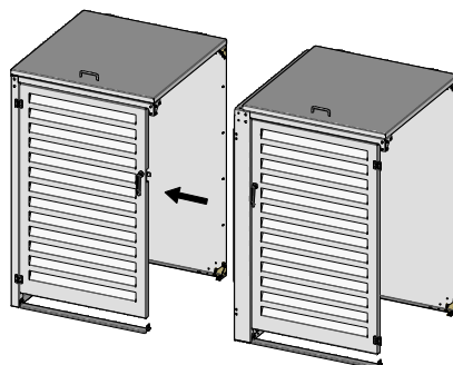
MODULE COMPLÉMENTAIRE (POUR 2e CONTENEUR) RÉFÉRENCE: MACMC240
