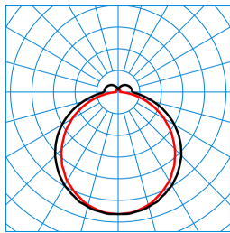
Olisq LWD2 DW 20-840 ET HFS IP54 IK TX430032
