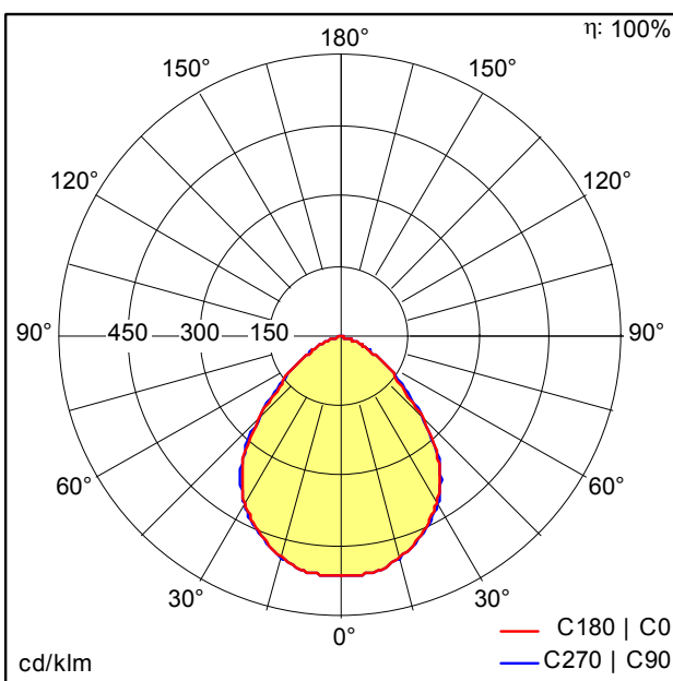
D46061_LF3_E_5000-940_M600L12_EVG.Idt
